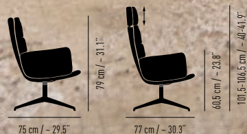
4-Fuß-Stern-Gestell SL, Sitzhöhe + 3,5 cm 4-leg star frame SL, seating height + 3,5 cm
