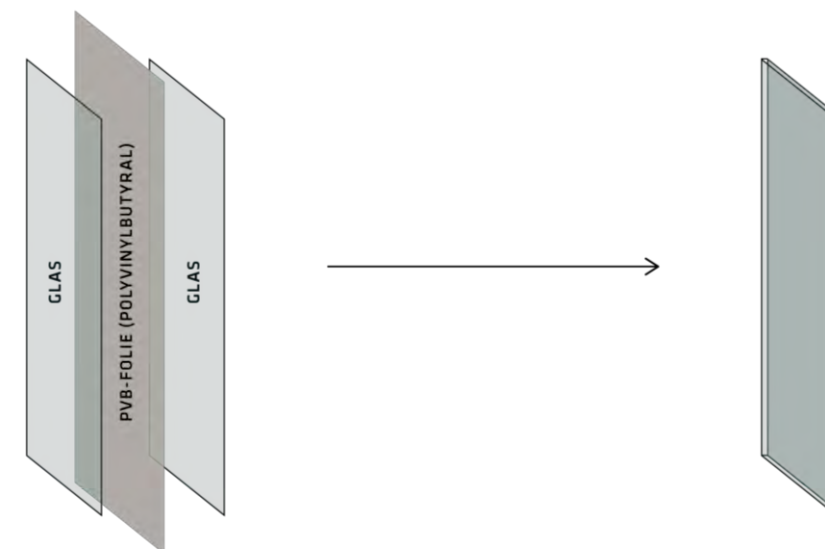
ZUSAMMENSETZUNG VERBUNDSICHERHEITSGLAS
